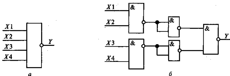
Рис. 4.6. Один из четырехходовых элементов комбинационной логики ( а ) и его реализация через двухходовые элементы ( б )
