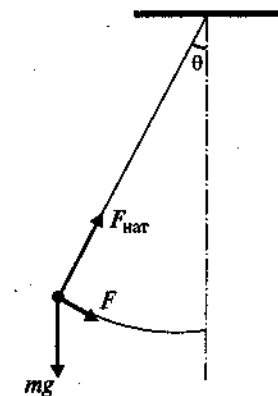
Рис. 7.4. Математический маятник
