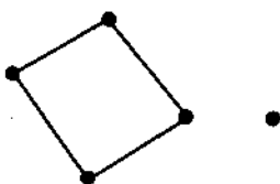
Несвязный граф
